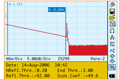
OTDR TRACE
